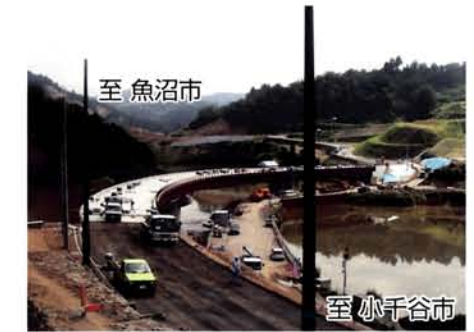
床版打設完了 平成18年8月10日
