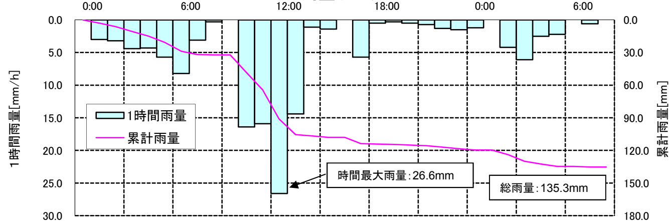
雨量データ
