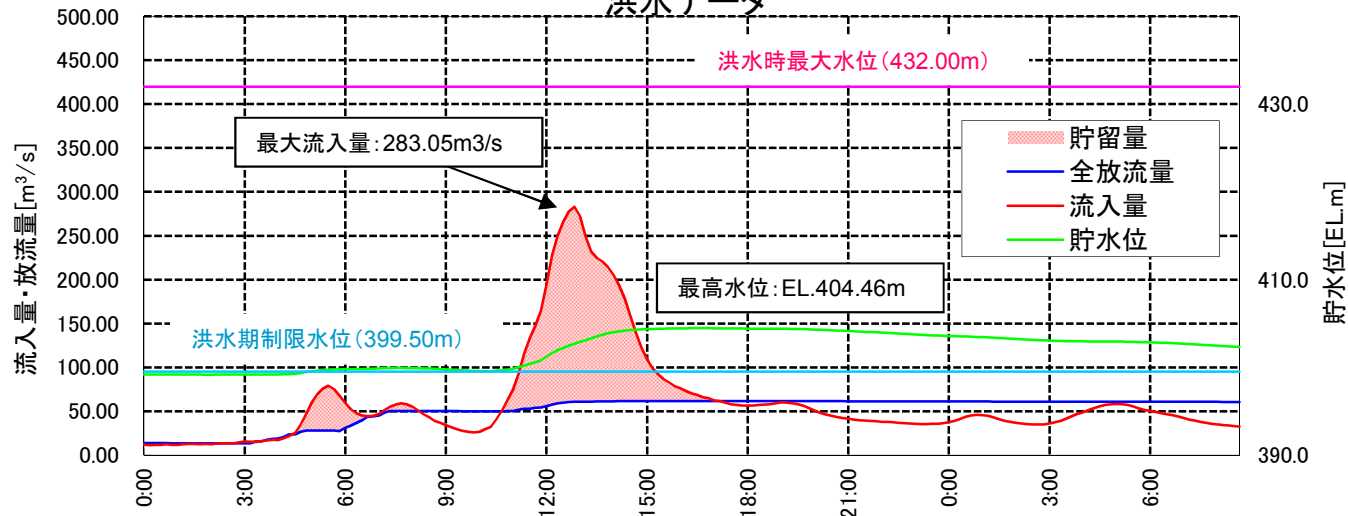
洪水データ
