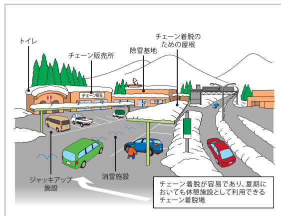
⑤多機能型チェーン着脱場
