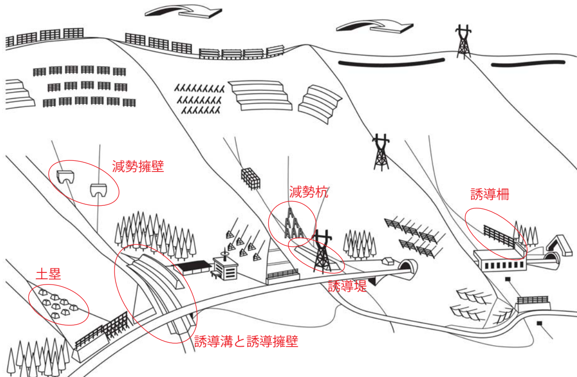
③減勢工と誘導工の役割
