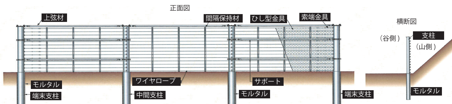
⑤せり出し防止柵の断面図
