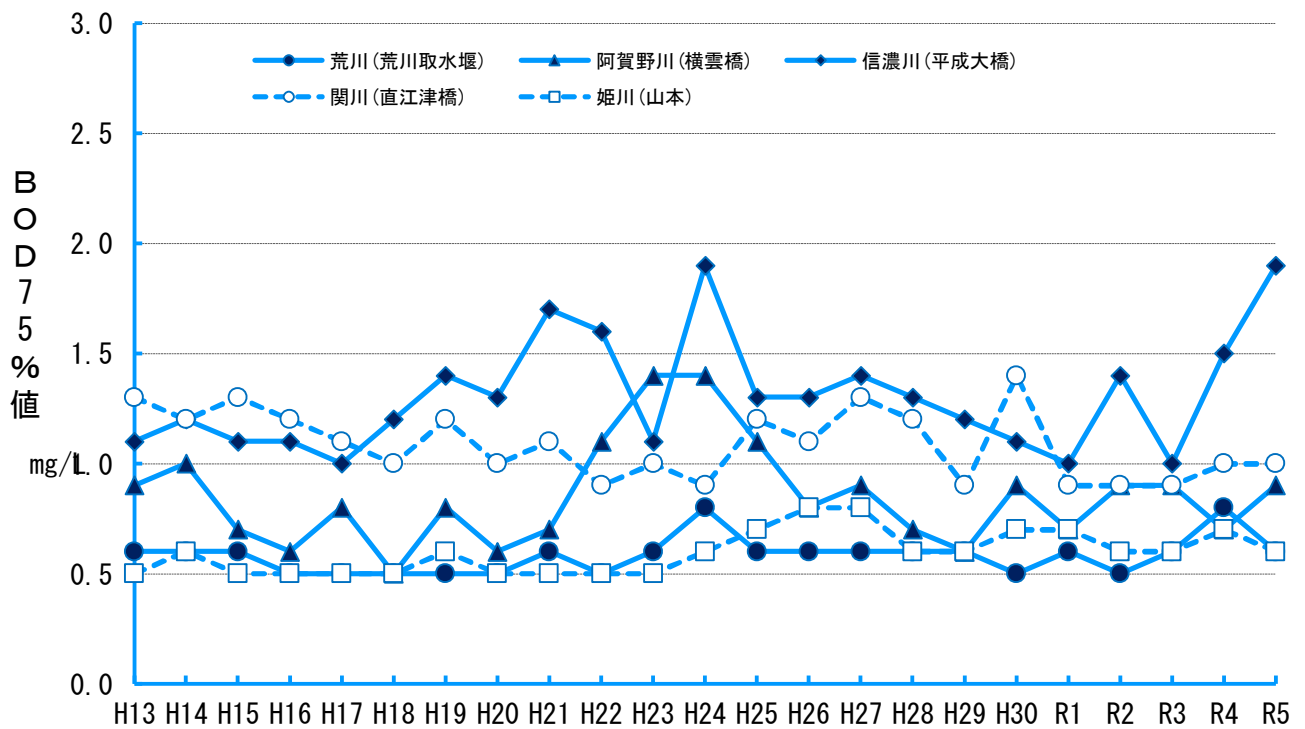
図－１－３ 主要河川の代表地点における水質の経年変化（その１）
