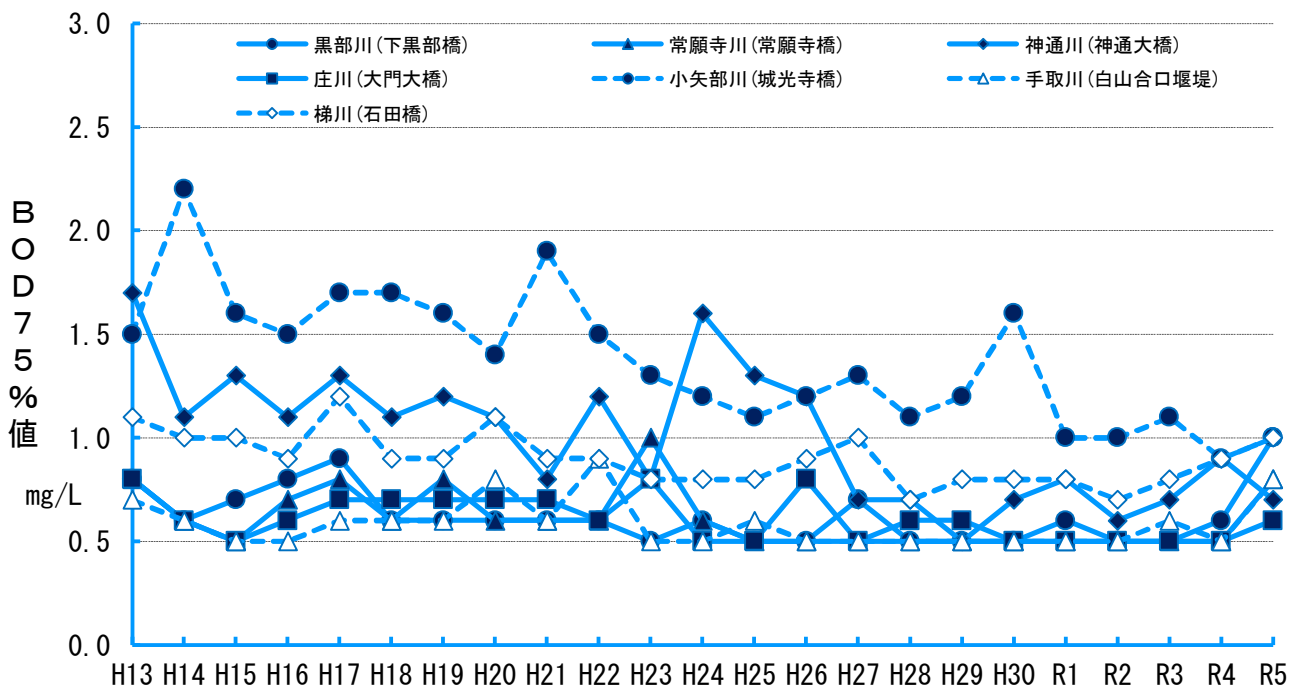
図－１－３ 主要河川の代表地点における水質の経年変化（その１）
