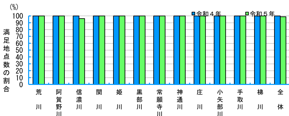
図-1-1 一級河川における環境基準値を満足している地点の割合経年変化
