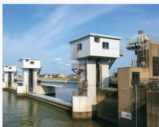
↑ 新潟大堰 (新潟県新潟市)
