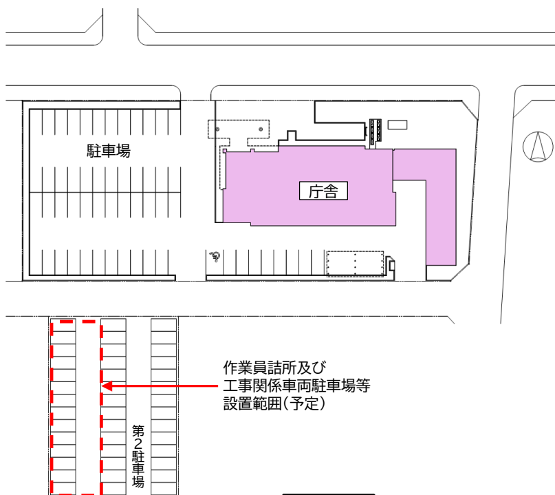
配置図
