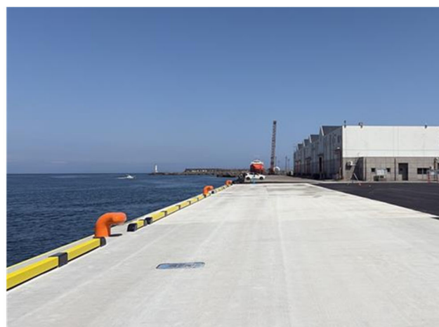
本事業で耐震改良した2号岸壁 （令和8年3月27日撮影）
