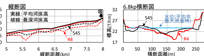
セグメント1 河川における河道の二極化進行の例
