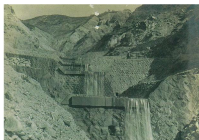
竣工当時の甚之助谷砂防堰堤群
