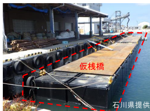
輪島港漁船だまり③仮棧橋設置状況 (6月26日)
