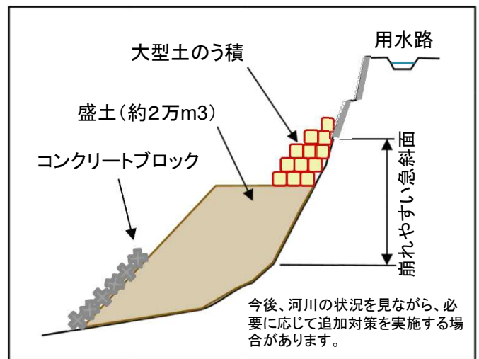
応急対策工のイメージ
