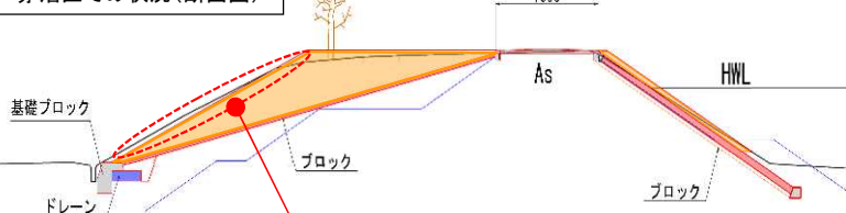
赤沼区での状況(断面図)
