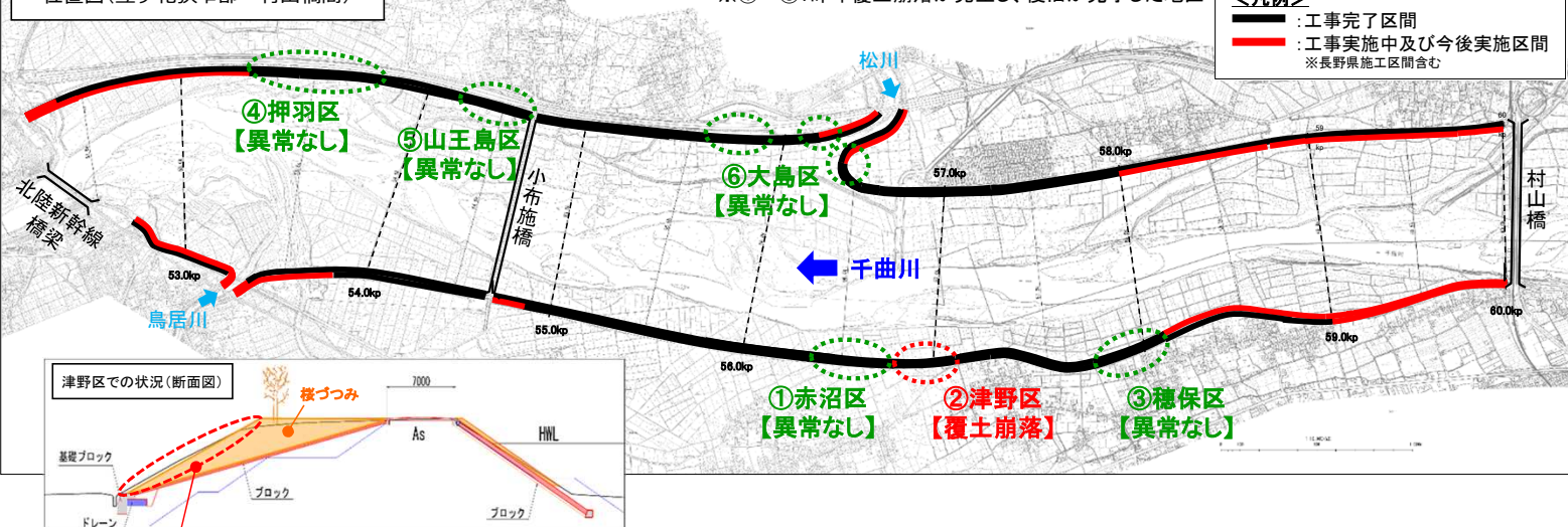
位置図(立ヶ花狭窄部～村山橋間)
