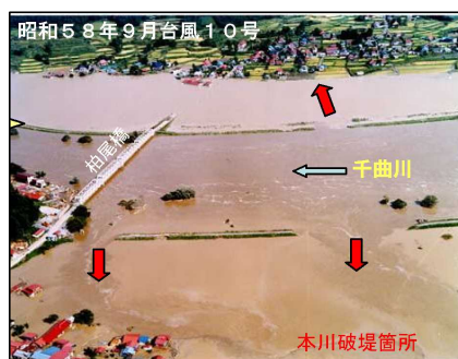
昭和58年9月洪水の被災状況 (飯山市照里地先)
