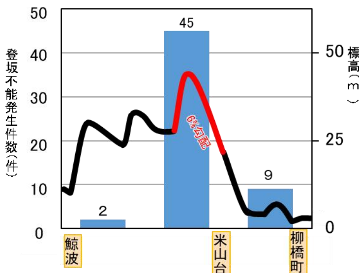
現道における登坂不能車発生状況 (集計期間: 平成20年～令和3年)
