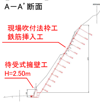
【断面図】
