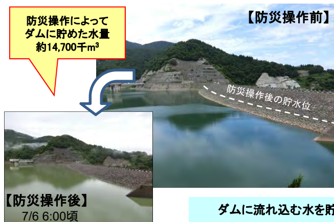
手取川ダムの貯水状況
