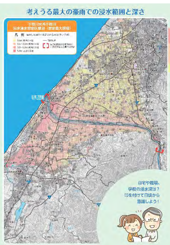
手取川浸水想定区域
