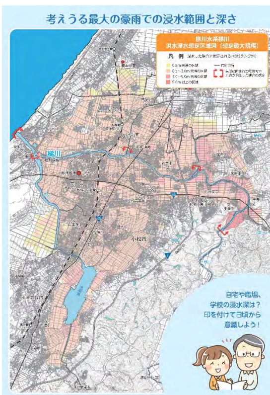
梯川浸水想定区域
