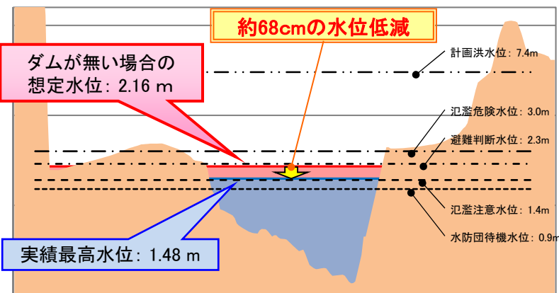
手取川の水位の状況 鶴来観測所地点
