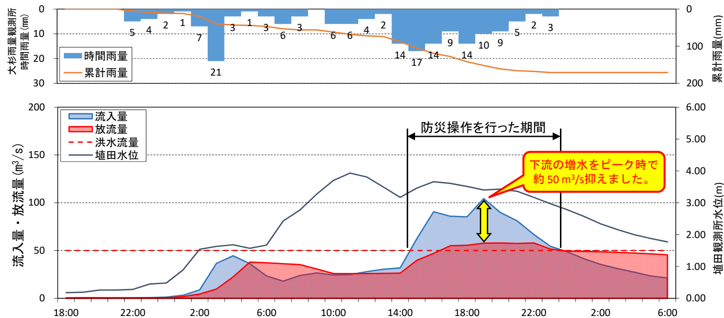
梯川の水位の状況 (埴田観測所地点)
