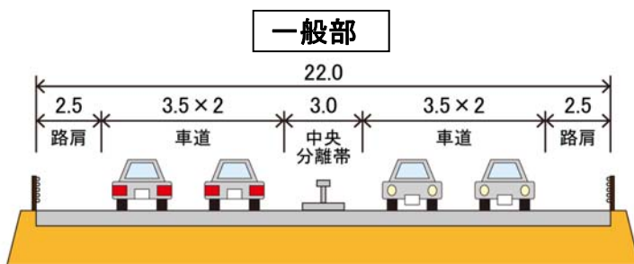
標準横断面図(完成4車線) (単位：m)
