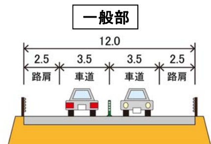
標準横断面図(暫定2車線) (単位：m)
