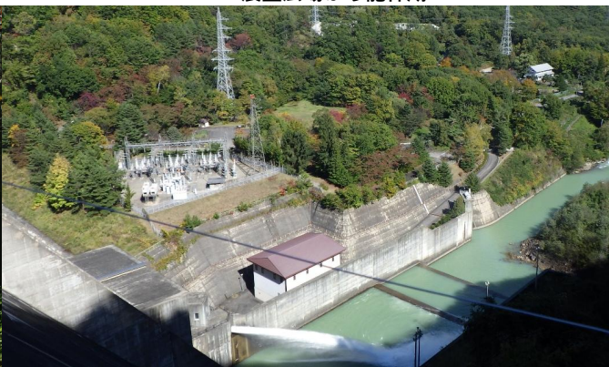
ジェットフローゲートからの放流
