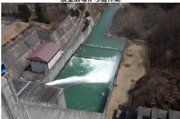
ジェットフロー放流②
