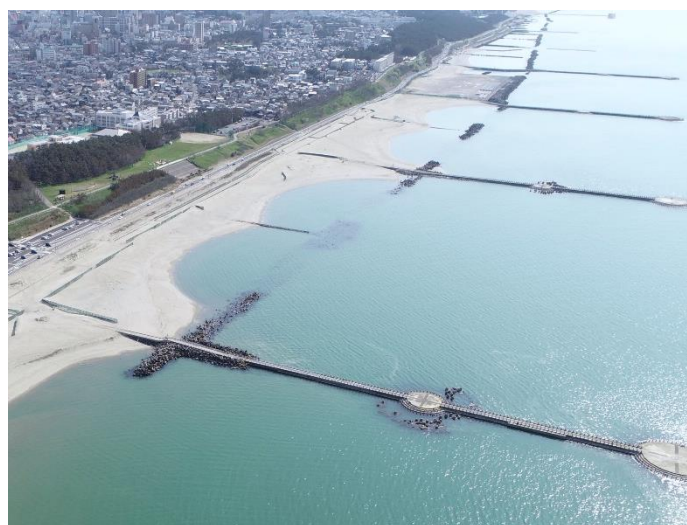
新潟の国土を守る、海岸の侵食対策（新潟市）
