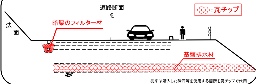
瓦チップ（53mm以下となるようチップ化）
