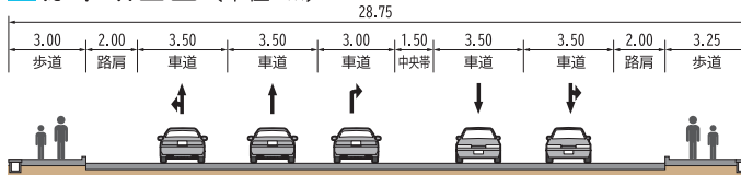
標準断面図 (単位: m)
