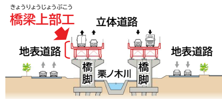
図. 橋梁上部工の範囲
