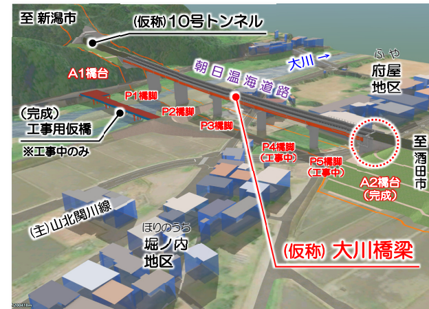
(仮称)大川橋梁 3Dモデル ※橋桁の色は未定です。
