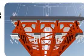
(仮称)大川橋梁 3Dモデル ※橋桁の色は未定です。
