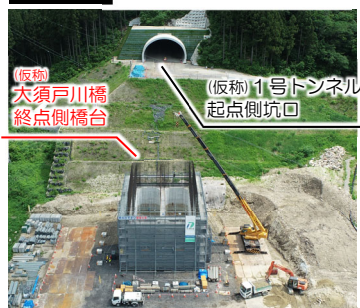
写真① (仮称)大須戸川橋
