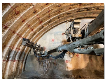
写真③ (仮称)11号トンネル
