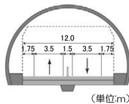
【標準断面図】
