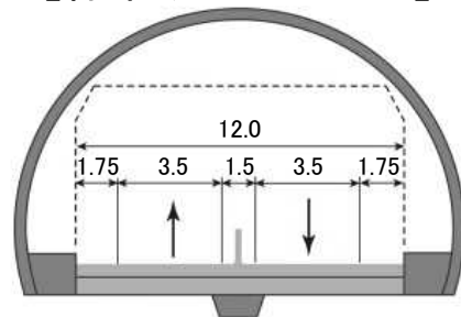
【標準断面図(単位:m)】
