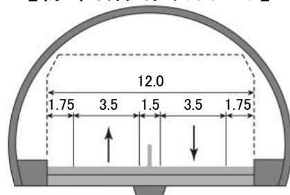
【標準断面図（単位：m）】
