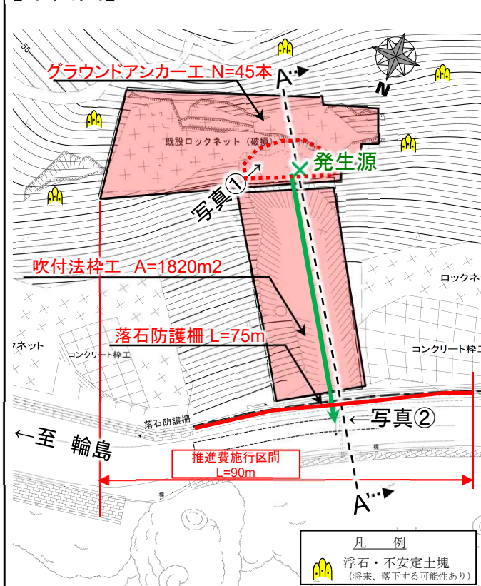
【平面図】
