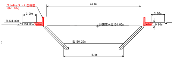
A - A'断面図
