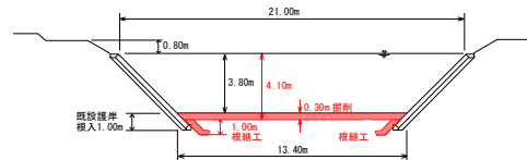
B - B'断面図
