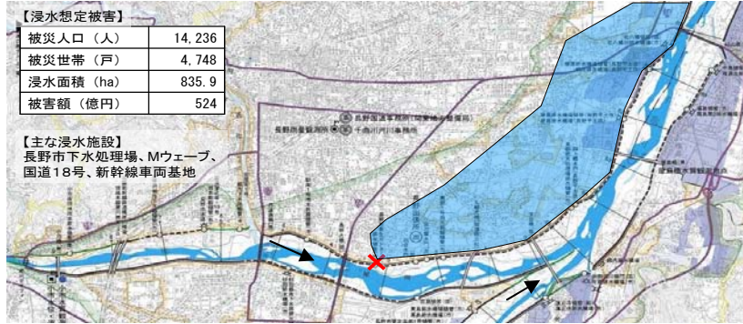
犀川左岸3.5k(長野市川合新田地先) 破堤時の浸水想定区域
