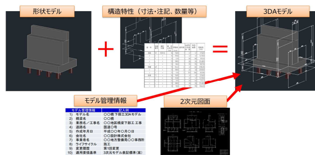
図-9 3DA モデルのイメージ 5)
