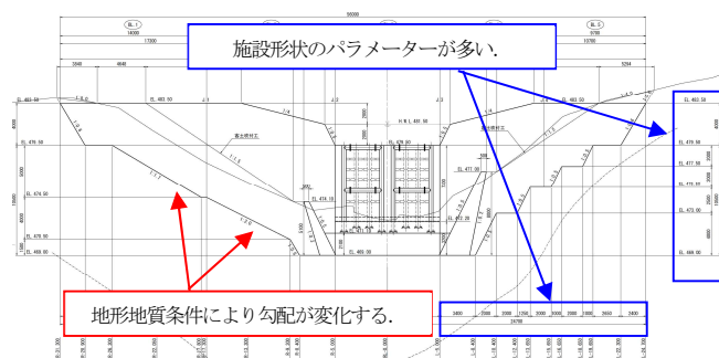
図-6 砂防堰堤正面
