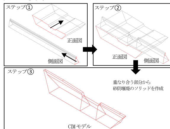
図-3 2次元図面からCIMモデルの作成例
