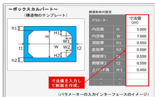
図-4 パラメトリックモデル 2)
