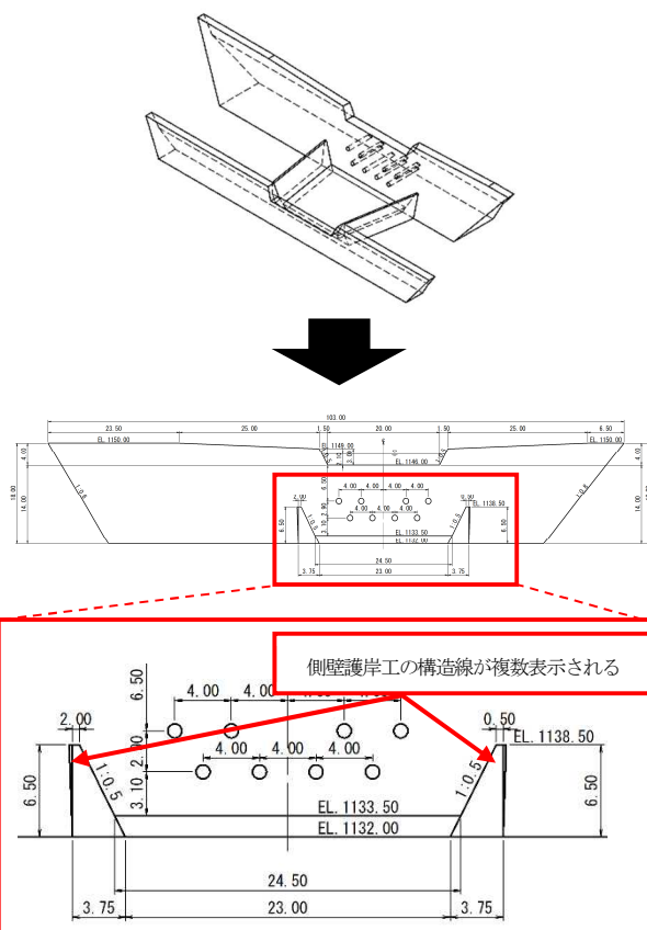
図-7 切り出しモデル
