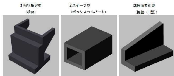
図-5 3次元モデルの特性に応じた使用 2)
