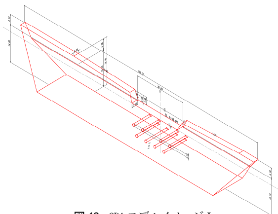
図-10 3DAモデルイメージⅠ
