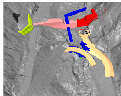
図-2 施工ステップ図 II
