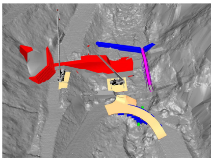
図-1 施工ステップ図 I
