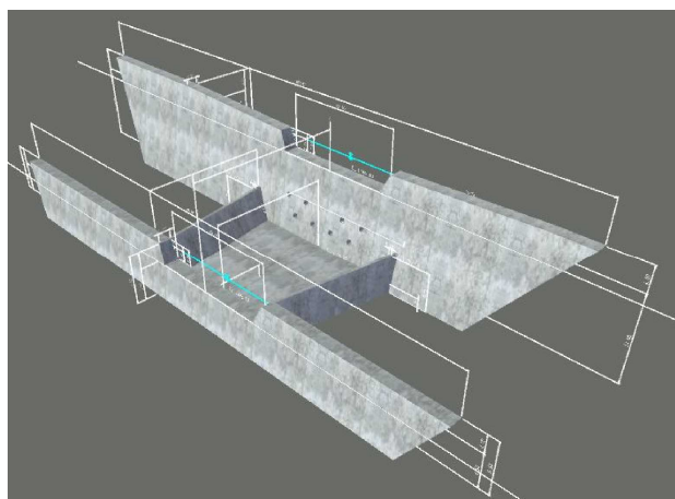
図-11 3DAモデルイメージⅡ
