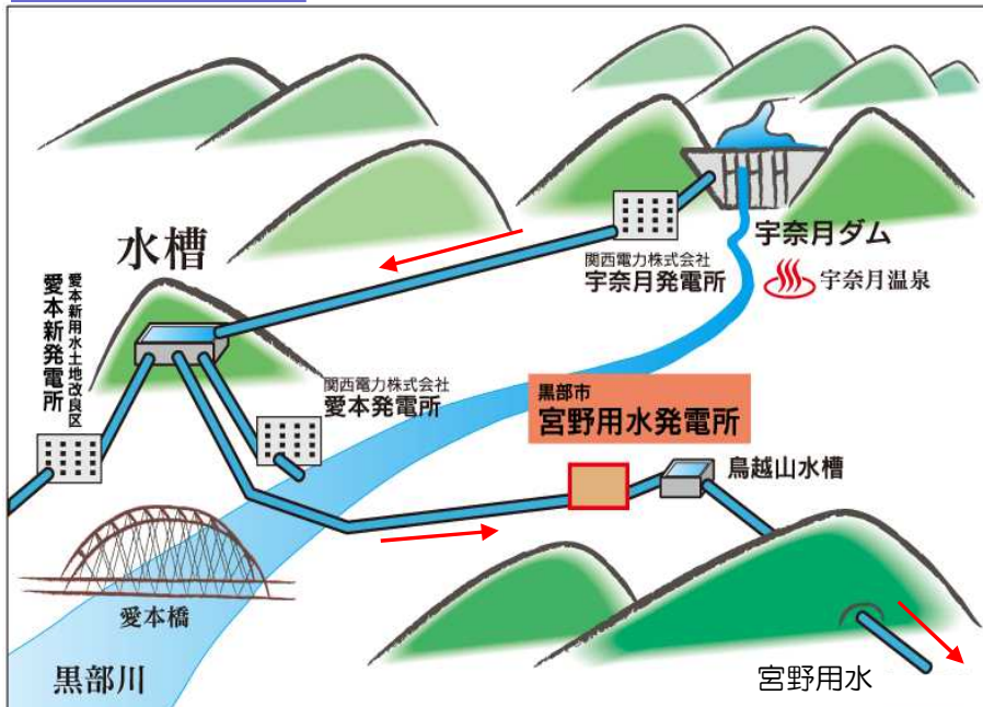
宮野用水系統図
