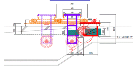
立面図
