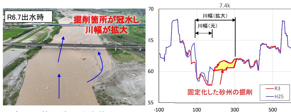
図2-6 施工前後の横断形状
