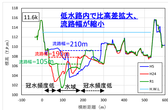
図2-2 流路幅と横断形状の経年変化(11.6k)
