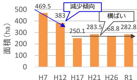
図2-9 礫河原面積の経年変化
