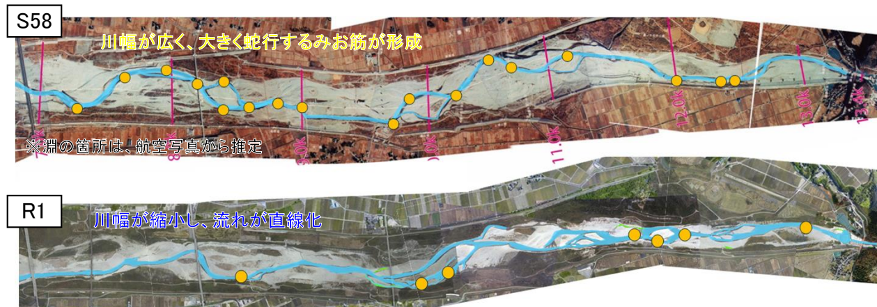
図2-3 みお筋と淵の数の経年変化(7k～13k)
