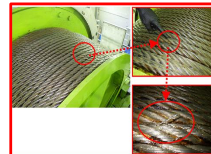
R07補正修繕予定 排砂設備 2号止水ゲート ワイヤーロープ取替
