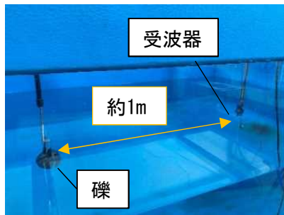
【水槽内の設置状況】
