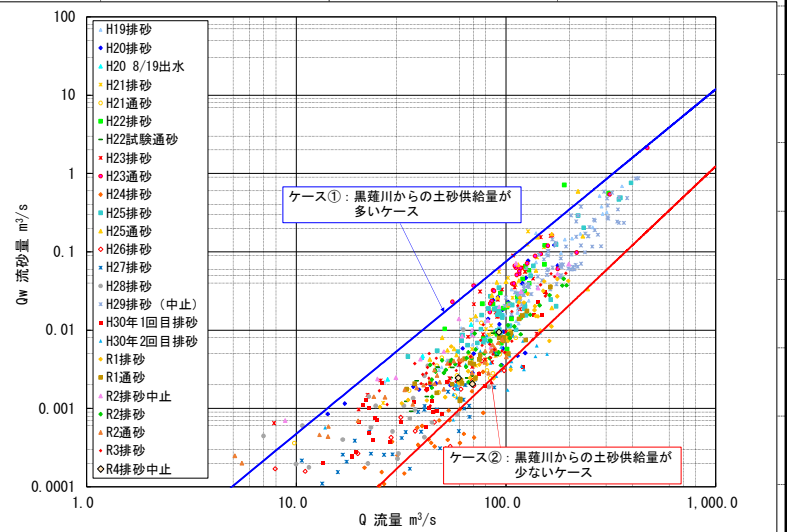
黒薙川より流入する土砂のうちSS成分の流量と流砂量の関係
