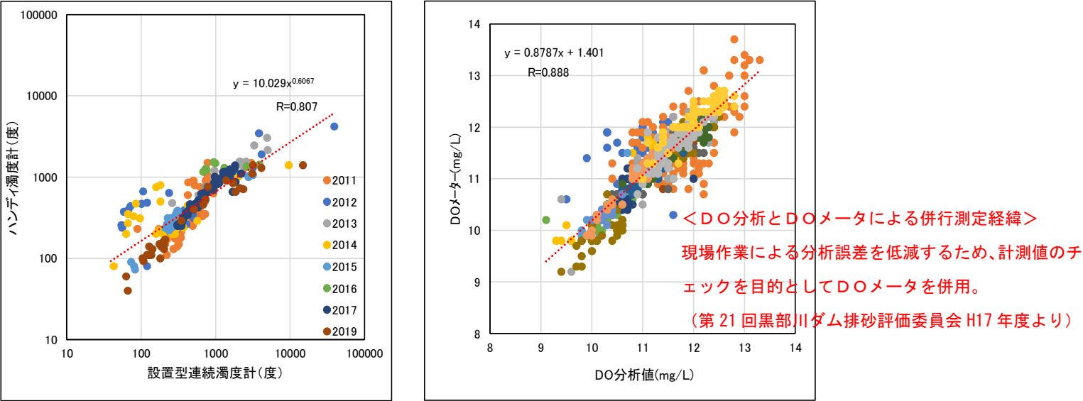
図 1.1-4 出し平ダム直下における設置型とハンディ濁度計の相関
