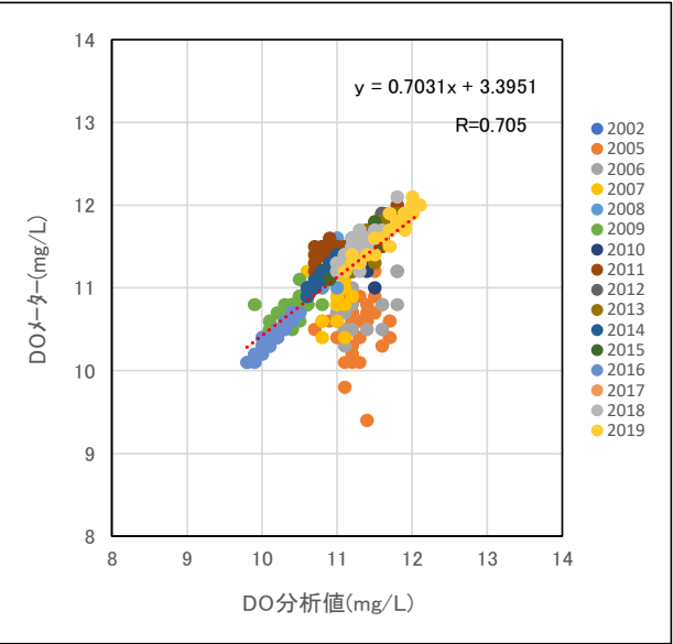
図 1.1-8 猫又における DO 分析値と DO メータの相関
