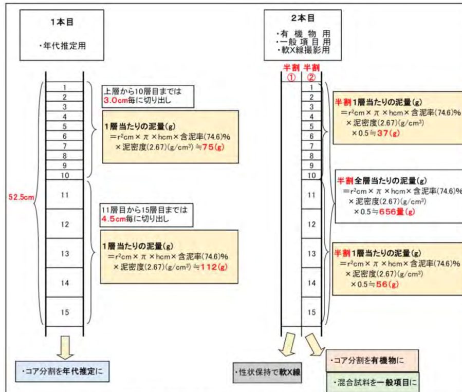
図 - 2 コアサンプルの調整方法（ピストン式柱状採泥器（小型）による場合）
