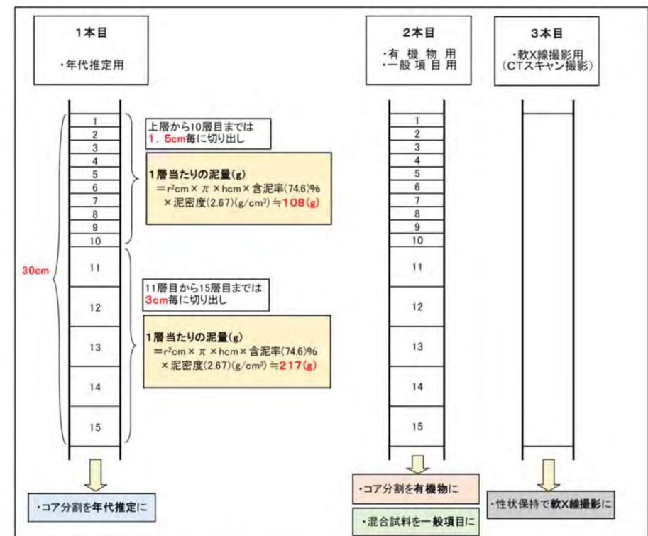
図 - 3 コアサンプルの調整方法（長尺アシュラ採泥器による場合）
