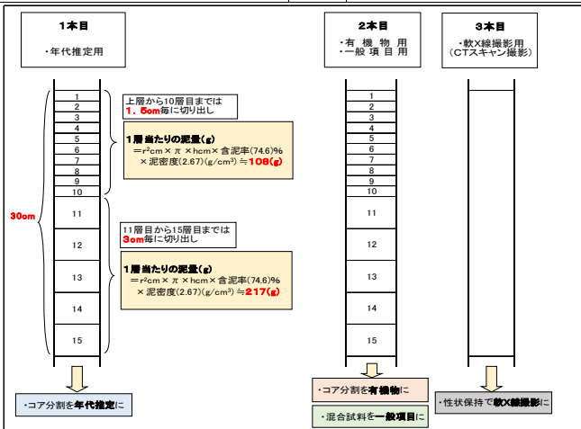
長尺アシュラ採泥器試料調整方法
