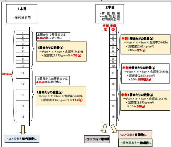
小型ピストンコアラ試料調整方法
