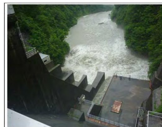
【出し平ダム下流】自然流下完了(EL.308.80m) 7月7日 8:50撮影
