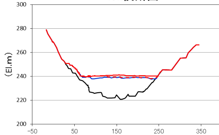
22.6k横断面図
