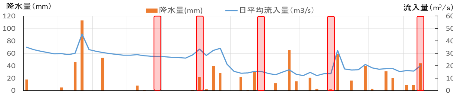
魚津における降水量と出し平ダムの流入量 出所: 気象庁ホームページ、関西電力データ
