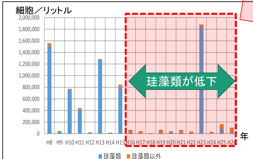
11月海域調査における植物プランクトン細胞密度の経年推移 (平成8年～26年、調査地点4点の平均値)
