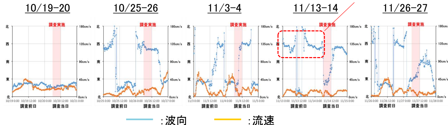
入善沖における波向と流速 出所: 富山水産研データ
