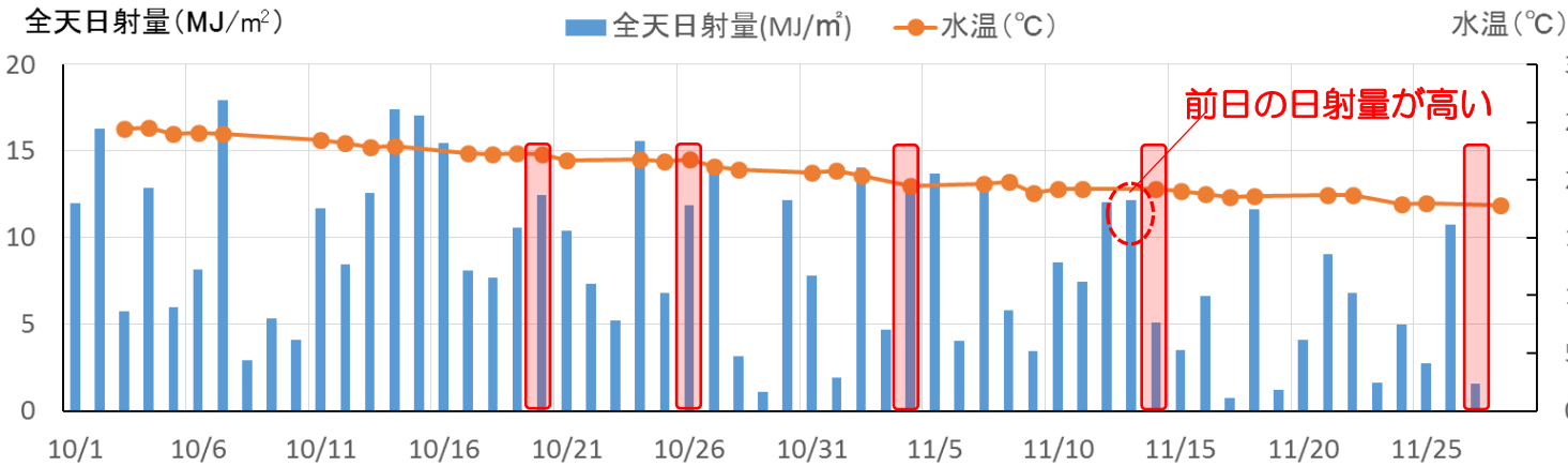
滑川における水温と富山における全天日射量 出所: 気象庁ホームページ、富山水産研データ
