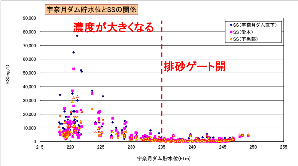
a)貯水位とSSの関係
