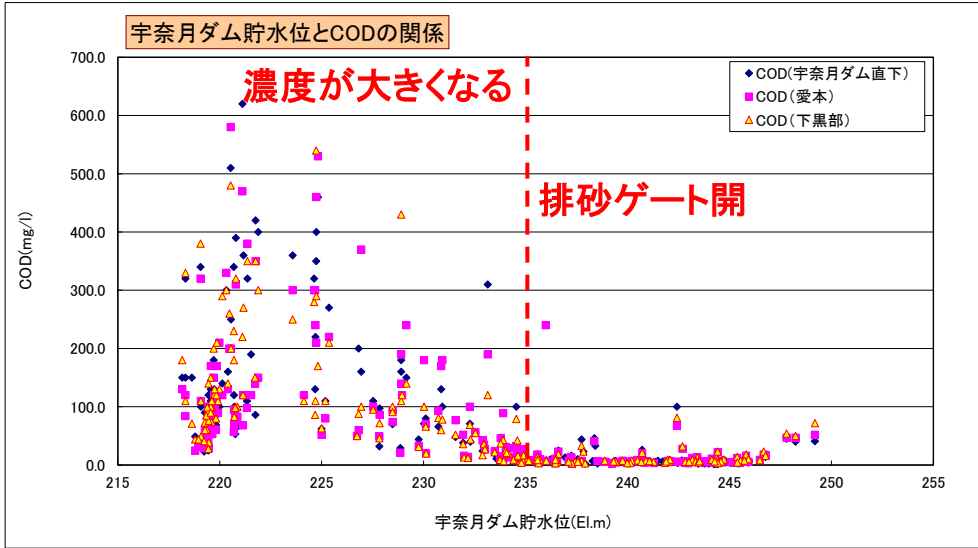
b)貯水位とCODの関係
