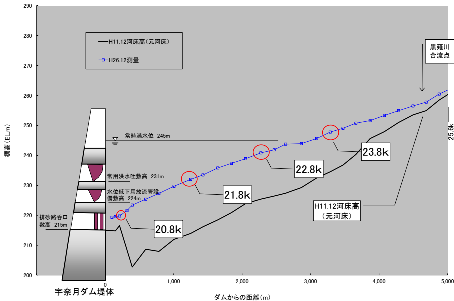
図-4.7 宇奈月ダム貯水池縦断面図
