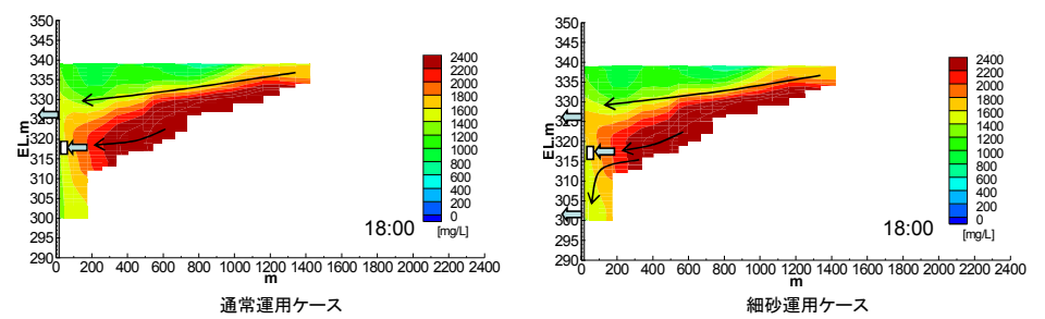
図3 放流SSシミュレーション結果(8/30)
