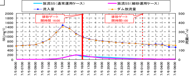
図1 放流SSシミュレーション結果(7/5)
