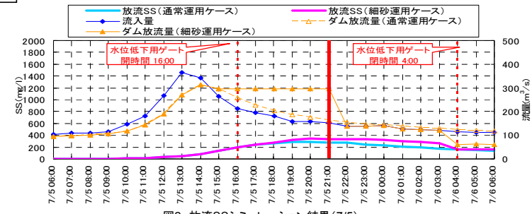
図2 放流SSシミュレーション結果(7/5)
