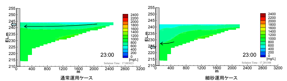
図4 放流SSシミュレーション結果(8/30)
