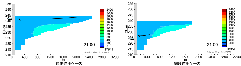
図2 放流SSシミュレーション結果(7/5)
