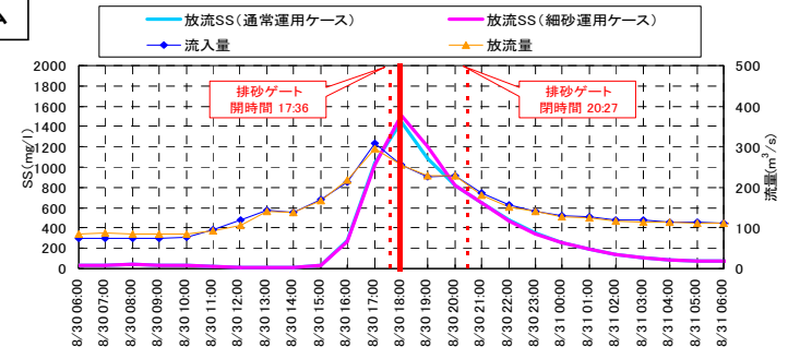
図3 放流SSシミュレーション結果(8/30)
