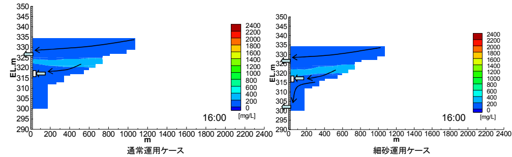
図1 放流SSシミュレーション結果(7/5)
