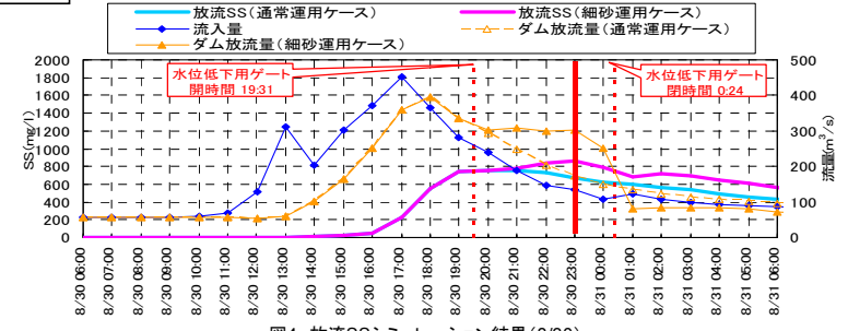
図4 放流SSシミュレーション結果(8/30)
