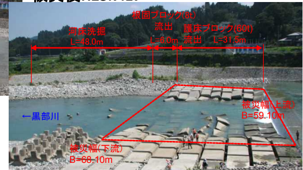
河床低下により被災した愛本床止め工
