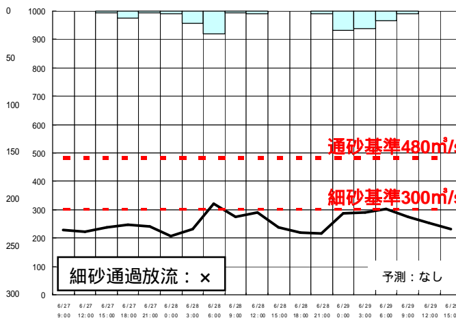
図1-2 第1回細砂通過放流実測流入量
