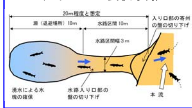
タイプ2：ブロック設置水路
